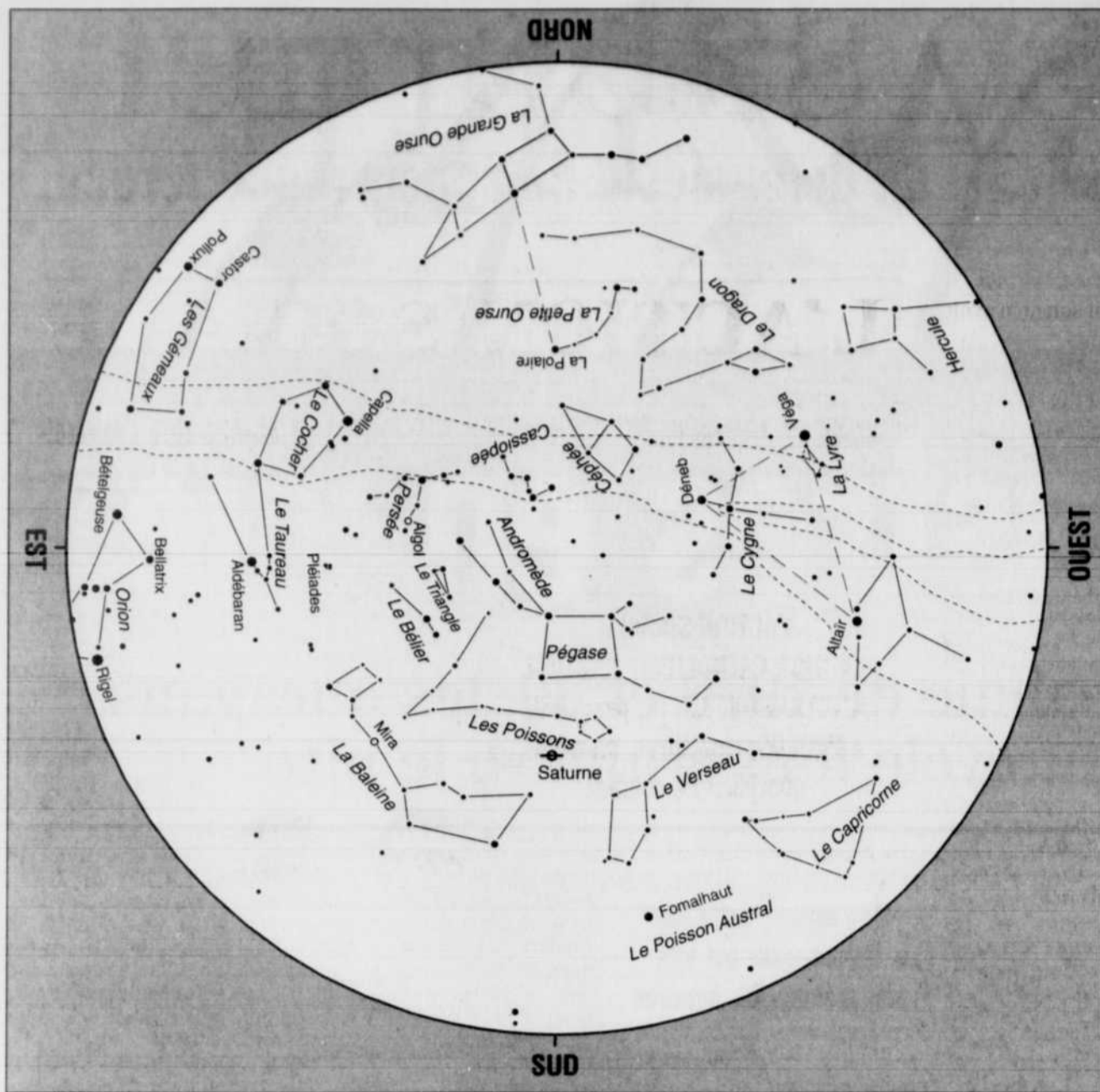
La carte montre l'aspect du ciel vers 21h30 (HNE) le 15 octobre (une heure plus tard au début du mois, une heure plus tôt à la fin). Pour l'utiliser, tenez la carte au-dessus de votre tête en alignant les directions avec les points cardinaux. Les lignes pleines montrent le contour des constellations, et les lignes pointillées ceux de la Voie Lactée.
