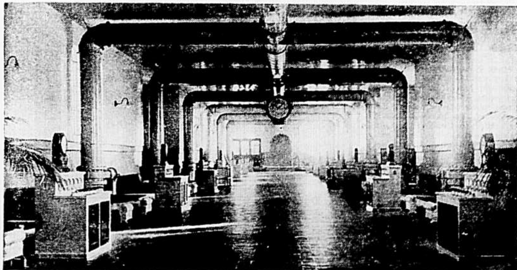
Une des galeries des lits de filtration. Chacune des boîtes de contrôle que nous voyons correspond à un bassin qui prend naissance directement en arrière de chacune d'elles pour s'étendre sur une longueur de 400 pieds. C'est là que l'eau passant au travers d'une couche de 30 pieds de sable et de 15 pouces de gravier s'égoutte dans le conduit qui la dirigera après chlorination vers le bassin d'eau filtrée.
