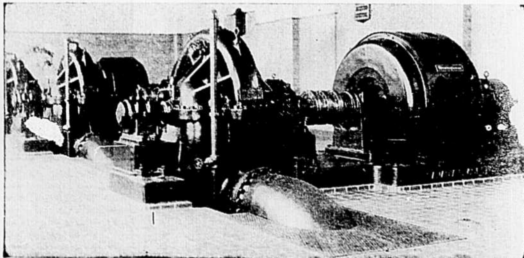
Ces pompes à haute pression, les plus modernes et les plus perfectionnées qui soient, pompent l'eau filtrée du bassin souterrain dans les différents conduits qui la distribueront dans toutes les parties basses de la ville et aussi au bassin d'eau filtrée de la station McTavish.
