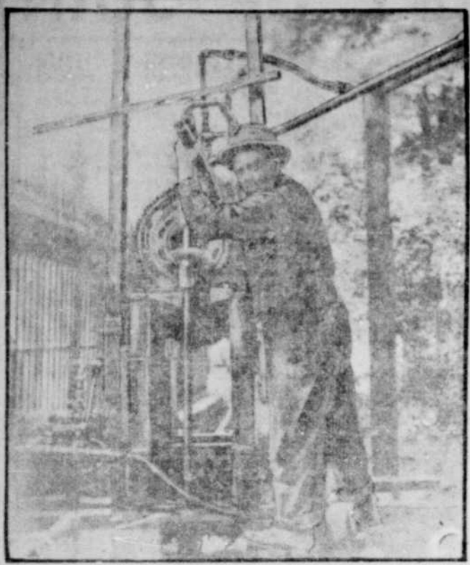
Depuis quelques jours, une équipe d'ouvriers sous la direction de la "Montreal Tunnel & Excavation Co." a commencé à creuser le tunnel de la ligne de chemin de fer de Dorchester et Saint-Monique.
