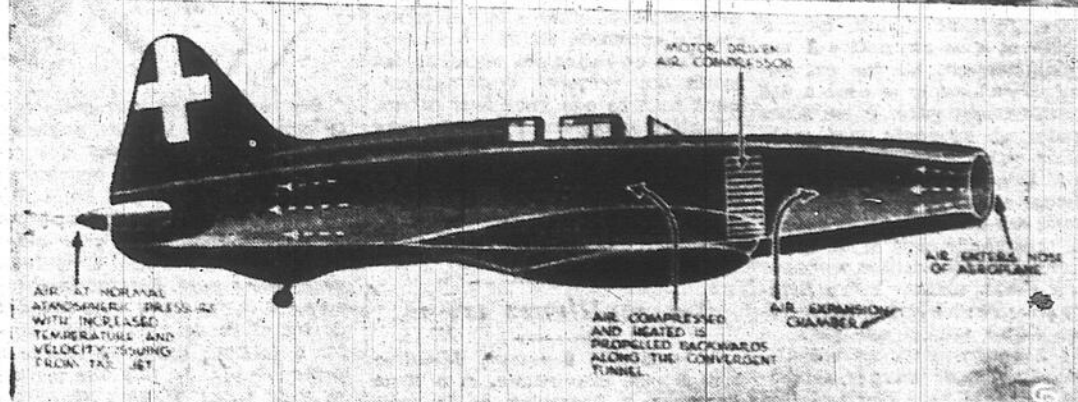
Le nouvel avion sans hélice de l'Italie, baptisé le "cigar volant" et l'avion "à air chaud", est montré et expliqué dans cette photographie et ce diagramme, grâce à la courtoisie de la revue anglaise "The Aeroplane". Cet aéroplane, le "Caproni-Campini C.C.-2" a été dessiné et construit par Secondo Campini. Il est actionné par un jet d'air rejeté en arrière de la queue de l'appareil. L'air entre à travers un conduit circulaire, à l'avant, est dilaté et passe dans le condenseur. L'air comprimé est chauffé et rejeté par l'arrière de l'appareil.
