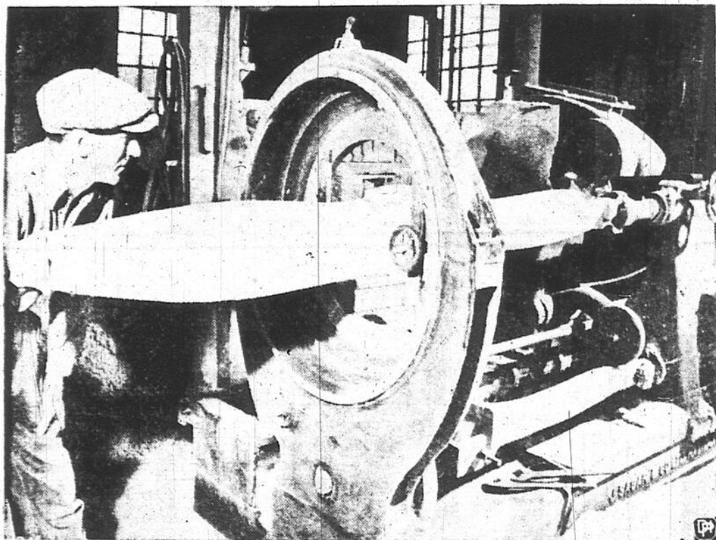
Une usine de Winnipeg où l'on construisait, avant la guerre, des traveaux mûs par des hélices aériennes, fabrique maintenant des hélices d'avions en bois laminé. Dans ce tour à profiler, les ébauches prennent rapidement la forme d'une hélice correspondant au modèle que l'on voit au bas de la machine. Ce tour accomplit en une demi-heure le même travail qu'un ouvrier mettait auparavant six heures à effectuer à la main.
