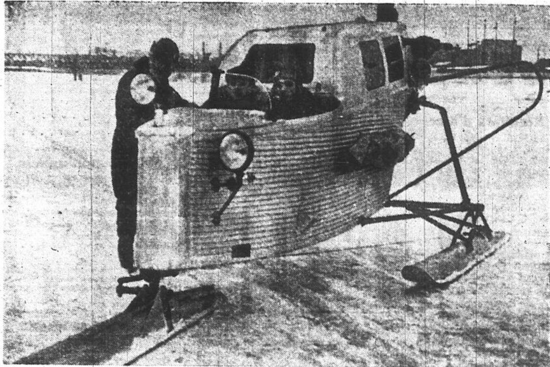
Construit tout en métal, ce nouveau type d'aéro-sleigh de l'armée russe a causé beaucoup d'ennuis aux soldats allemands les harassant de partout, aux endroits où les lourdes pièces mécaniques du Führer ne peuvent passer sans s'enfoncer dans la glace. Ces aéro-sleigh ont joué un grand rôle pour permettre aux Russes de reprendre la ville de Mozhaisk.
