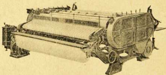
Calandre "Beaver" à 4 rouleaux.
