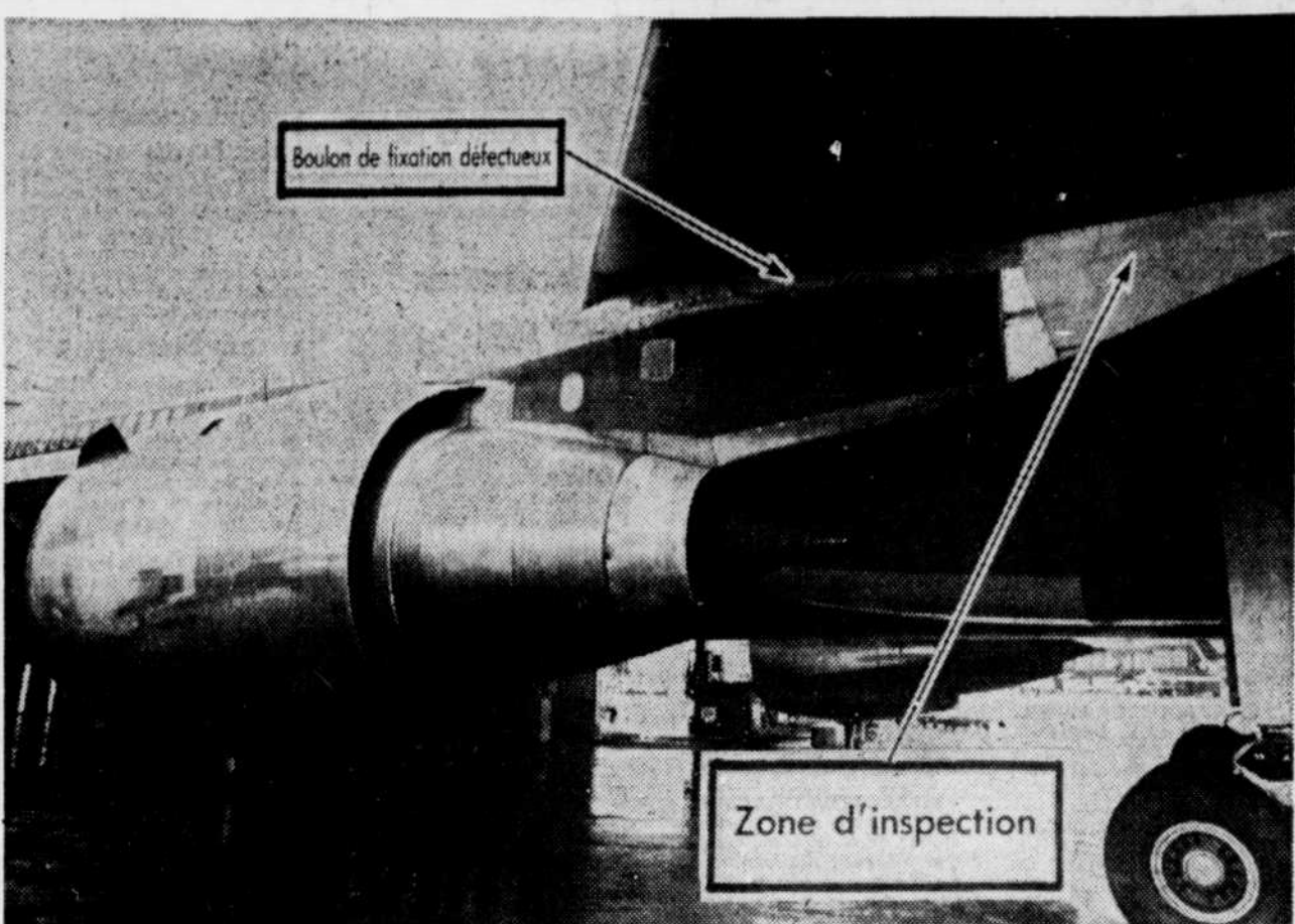
Immobilisé par mesure préventive, les DC-10 subiront une inspection minutieuse du système de fixation des moteurs. La flèche de gauche indique la position du boulon dont le bris a provoqué la tragédie de Chicago. La flèche de droite indique l'ensemble de la zone de fixation que le gouvernement américain ordonne de vérifier.
