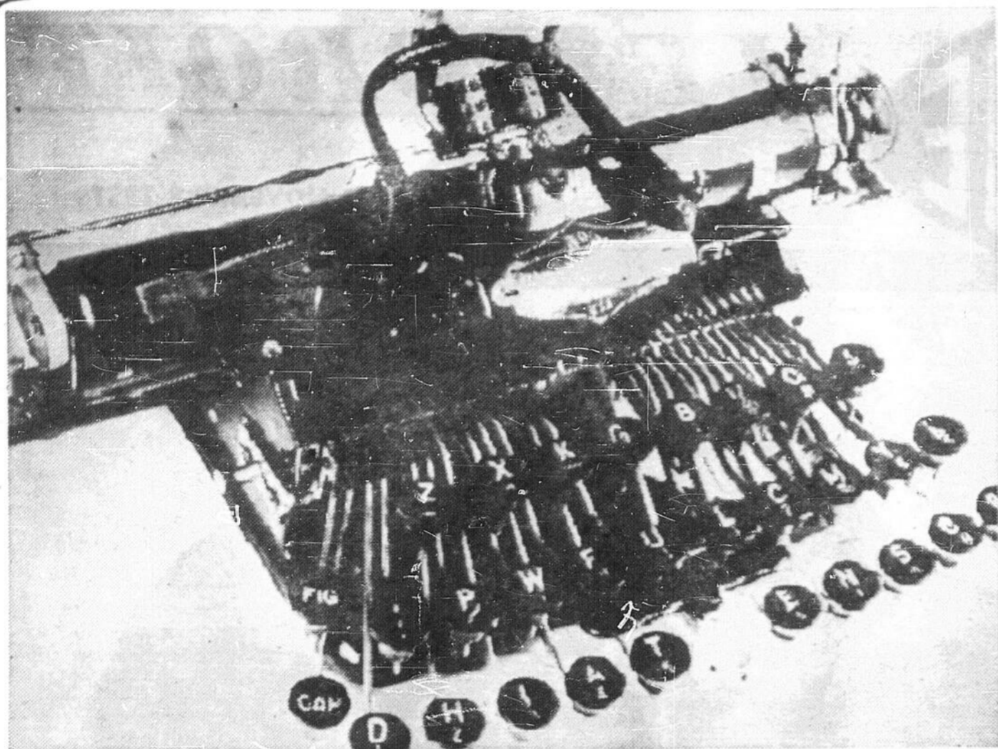
Voici le fameux dactylographe Blickensderfer de 1855. Cette machine était une véritable innovation pour l'époque puisque l'on pouvait lire entièrement ce que l'on écrivait. Le fonctionnement de l'appareil était assez simple puisque un rouleau-imprimeur touchait à un rouleau rempli d'encre avant de se rendre au rouleau où se trouvait la feuille de papier qui recevait les caractères.
