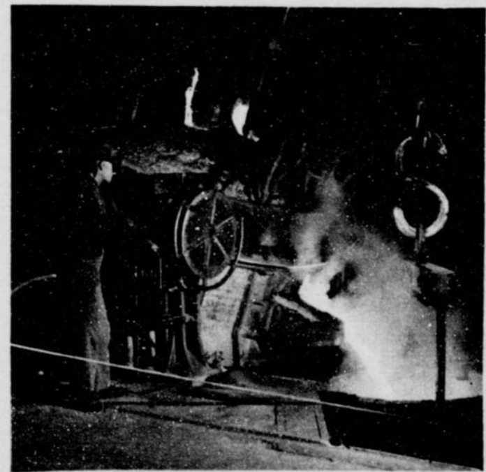
L'une des premières opérations de la fabrication du canon consiste à faire fondre la ferraille dans des fours dont la chaleur atteint près de 2,000 degrés. On trouve plusieurs fours de ce genre aux usines de Sorel
