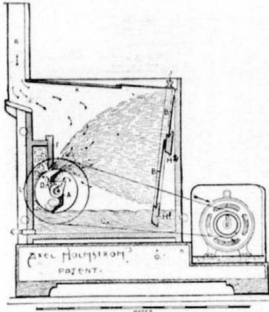
MACHINE À GRAVER.
