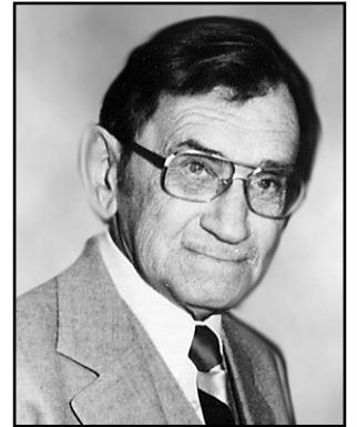
André Enault
