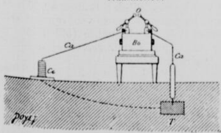
Schéma de l'installation du télégraphe sans fil par la terre (système Pilsoudski)
