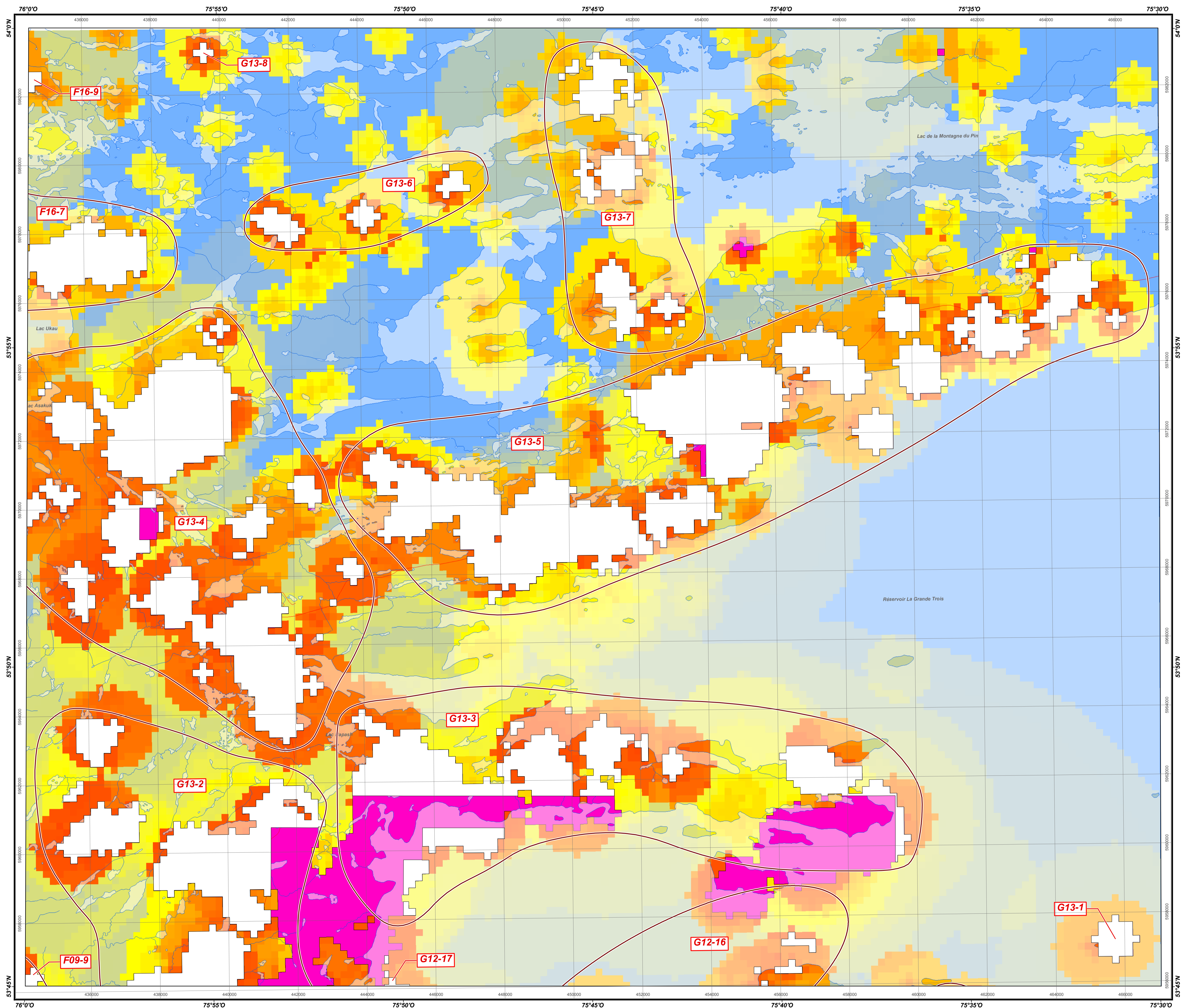
Carte d'évaluation du potentiel minéral pour les gîtes porphyriques de Cu-Au ± Mo de la Baie-James
