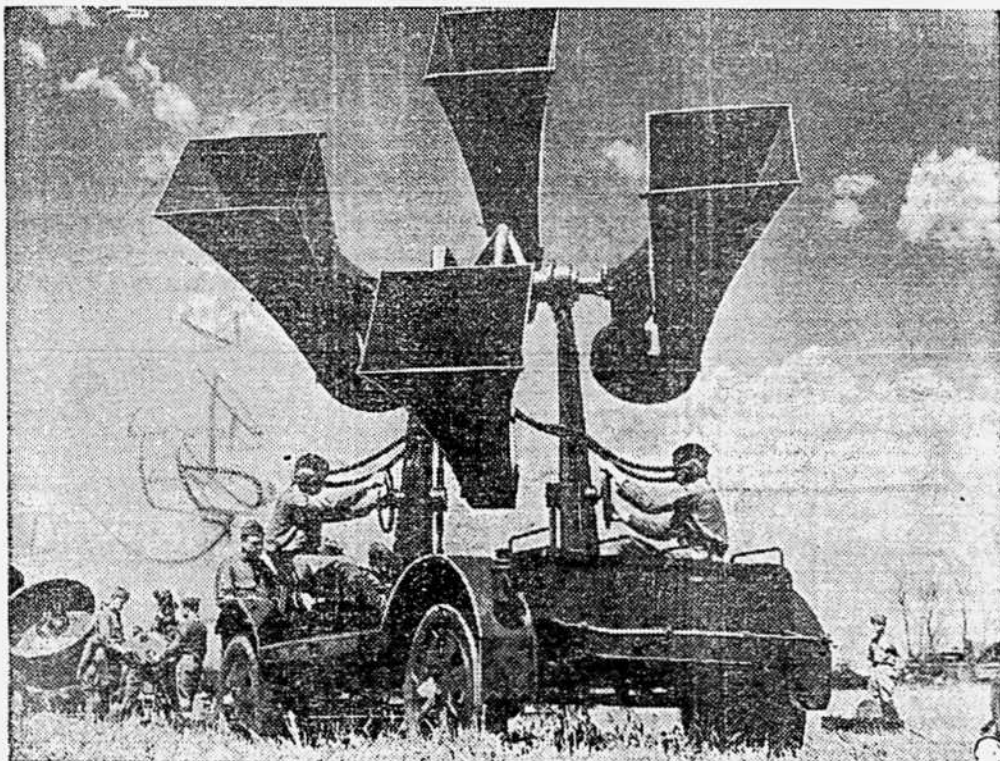
Un nouveau type de localisateurs pour le son qui constituent les "oreilles" au moyen desquelles on prévient les raids aériens.
