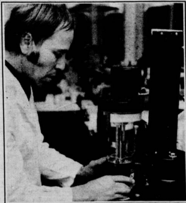
Le chimiste M. Chavigny des laboratoires Edith Serei soumet ici au visomètre une émulsion qui sert à la préparation d'un produit de beauté hydratant. Il faut que le produit soumis à l'expertise rencontre le plus parfaitement possible une foule de conditions d'hygiène et autres.
