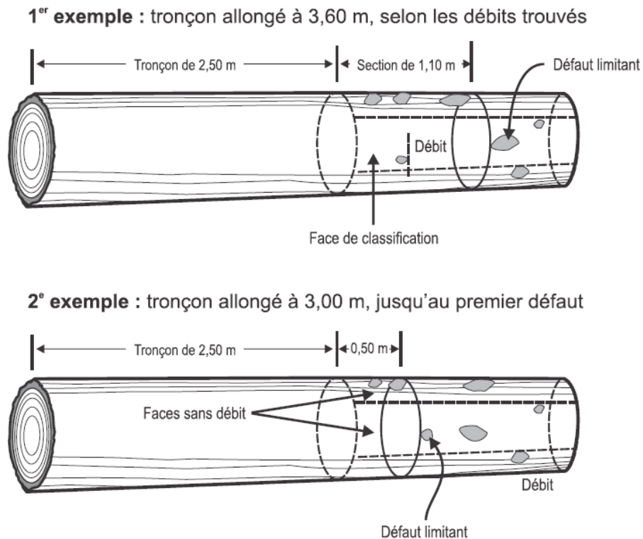
Figure 90 – Procédure pour allonger un tronçon selon les débits
