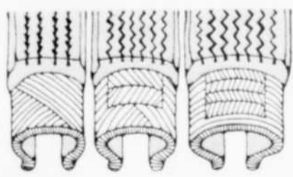
Carcasse ordinaire, Carcasse ceinturée, Carcasse radiale.
