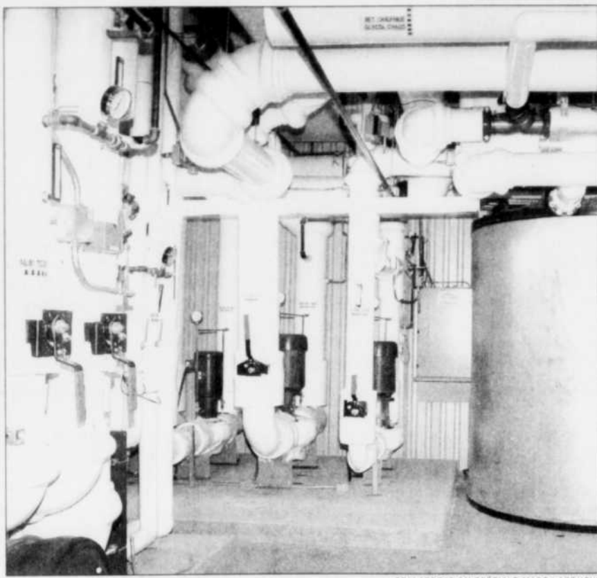
Ces immenses réservoirs sont des banques de glace. Le froid généré y est recyclé pour déshumidifier l'air du Centre Premier-Tech.
