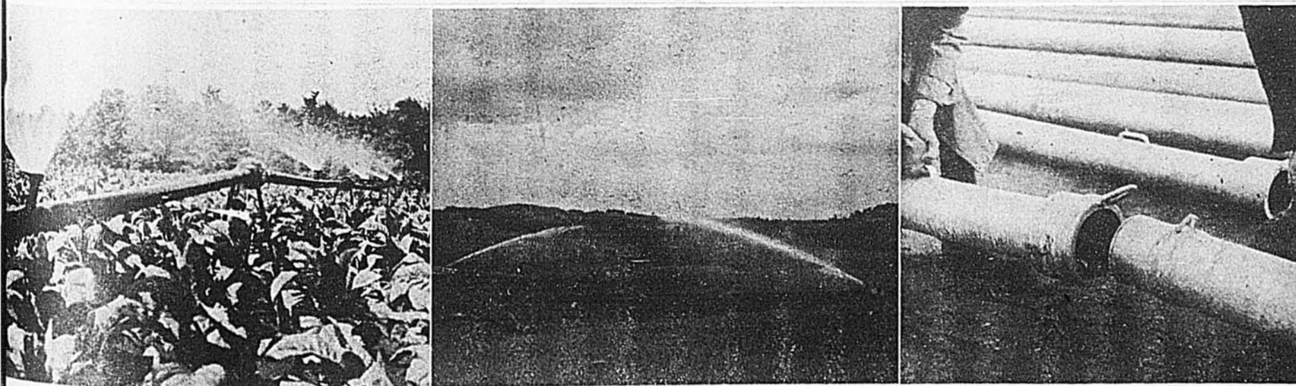
Ces trois photos, prises chez M. Robert Daigle de Warwick, Qué., illustrent bien de quelle façon ce cultivateur pratique l'irrigation. Sur la photo de gauche, l'eau est distribuée au moyen de jets: les tuyaux peuvent être déplacés, permettant ainsi d'irriguer une grande étendue de terrain. Au centre, c'est l'irrigation par tourniquets. Tel que l'illustre la photo de droite, les tuyaux dont se sert M. Daigle s'adaptent facilement les uns aux autres. Ce dernier système est démontable et le poids léger des tuyaux en facilite le déplacement.
