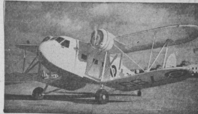
Originairement fabriqué pour combler le rôle d'un pilote de brousse comme transport de fret dans le grand nord, ce frétier Fleet est maintenant affecté au transport des cas d'urgence à l'hôpital du C.A.R.C. de Trenton, Ont. C'est un biplan à ailes doubles. L'appareil est peint en un blanc éblouissant, coupé d'une croix rouge sur les deux côtés du fuselage.
