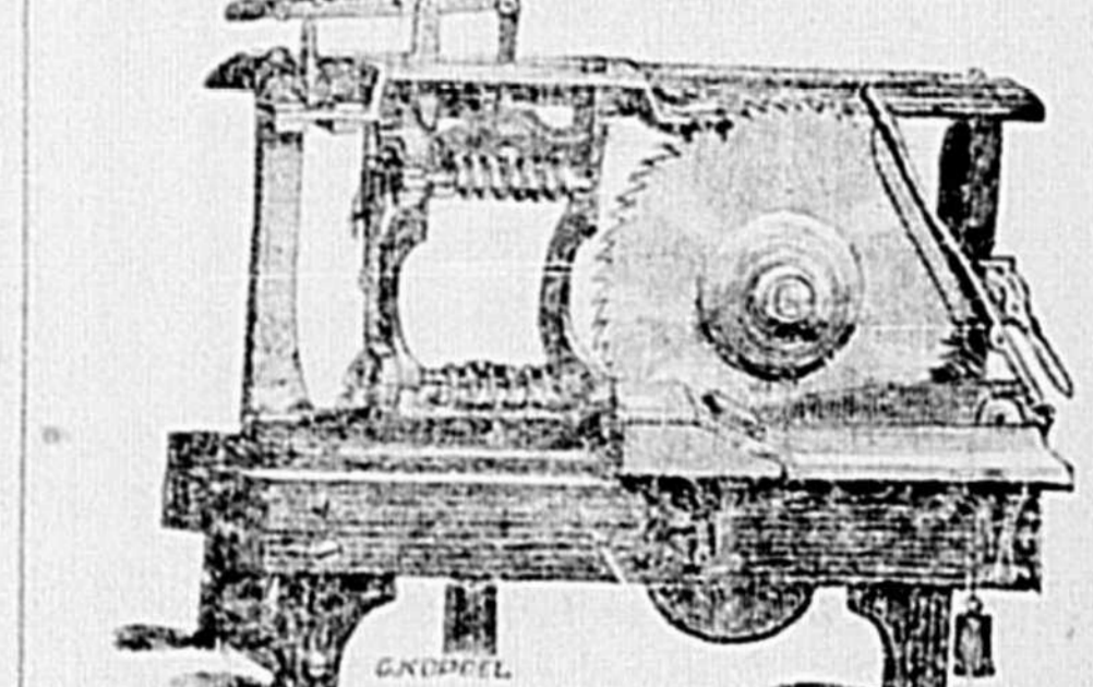
LA MACHINE BARDEAUX COMBINÉE Scie avec Planeur Redresseur
