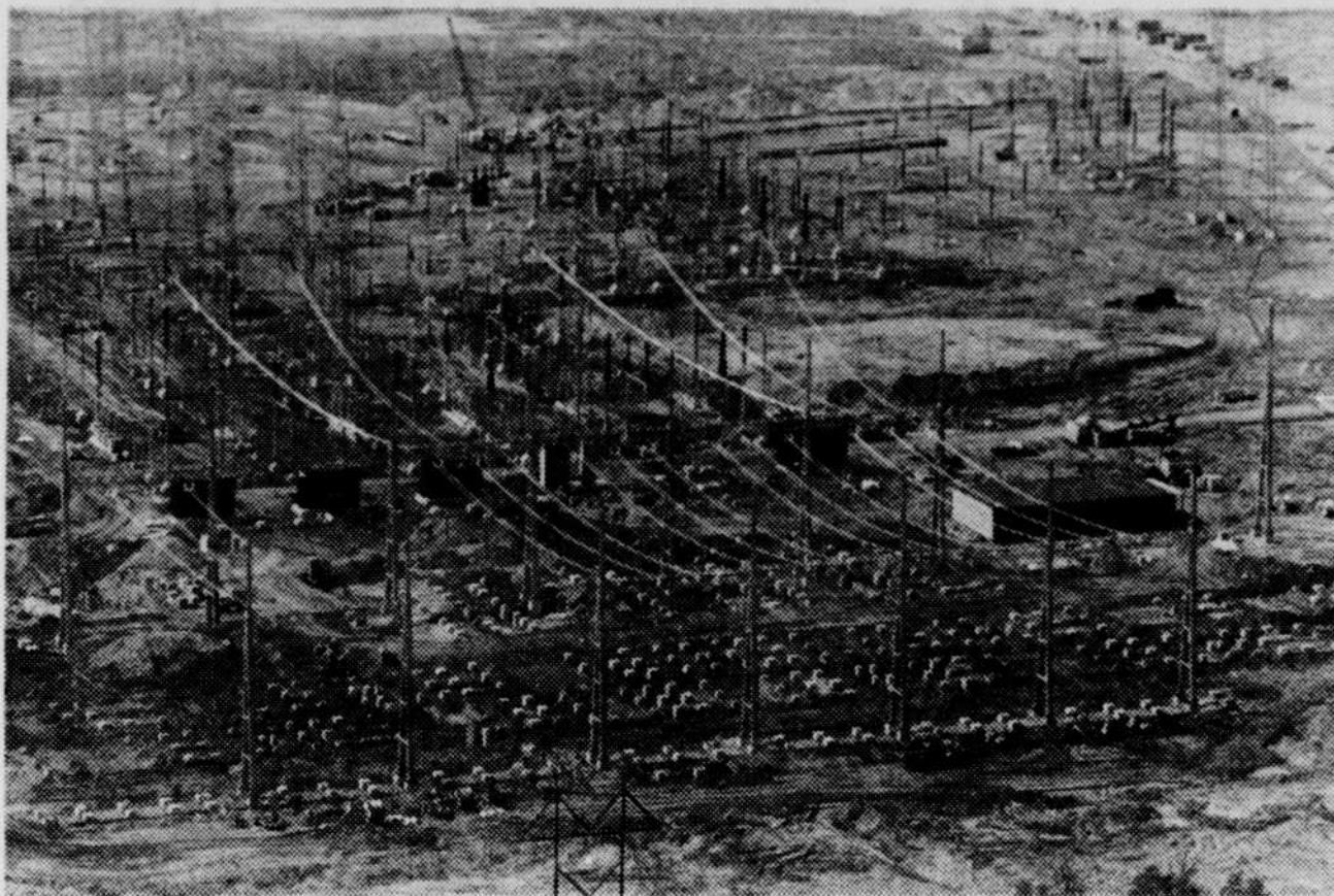
La vue aérienne sur le poste Nicolet, que l'Hydro-Québec construit au coût de $8,000,000, à Sainte-Eulalie, fournit une bonne image de la dimension et de l'importance du chantier. Au centre, on peut distinguer quatre des six transformateurs géants qui alimenteront le poste. L'ouverture du poste, d'abord prévue pour septembre, est retardée au début de 1974. (Photo Bo-Soleil)
