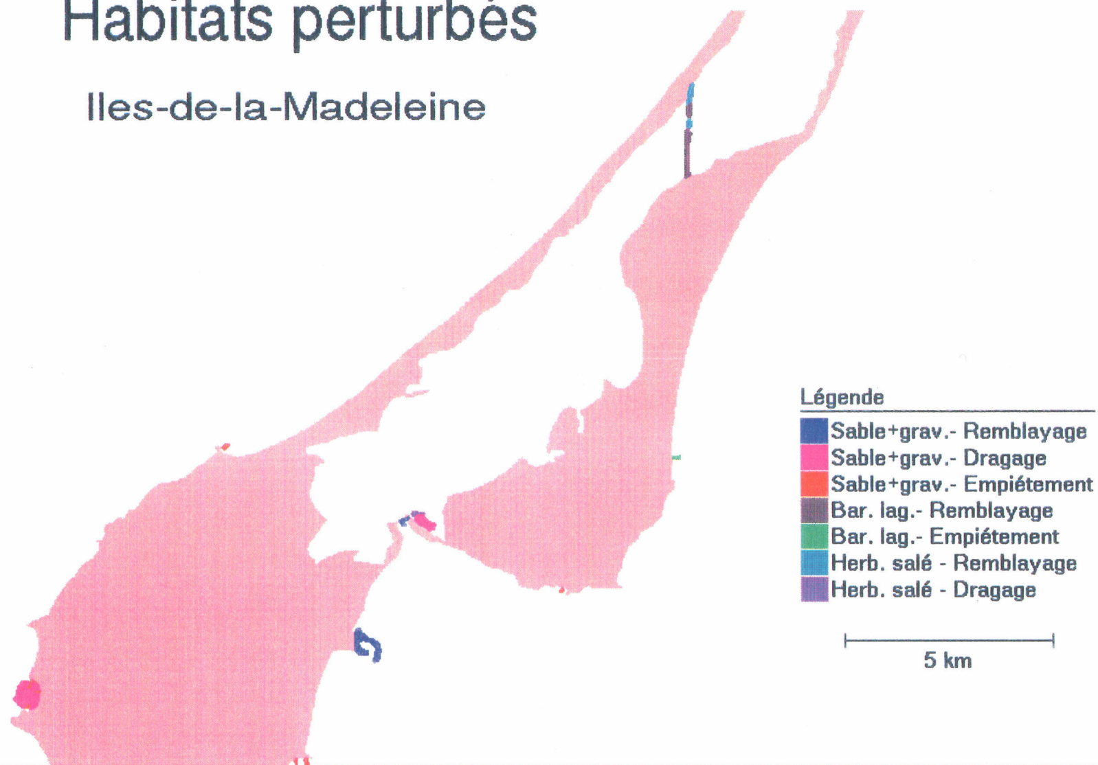
Figure 2.7 Habitats perturbés aux Îles-de-la-Madeleine (partie centre de la région)
