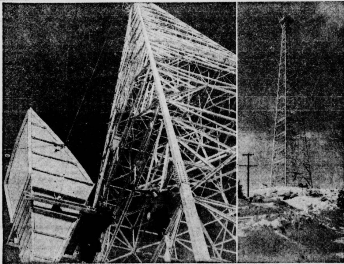
UNE ANTENNE GEANTE, pesant 1,900 livres, est hissée le long du pylône le plus élevé du réseau de relais radiotéléphoniques que construisent actuellement les membres du Réseau Téléphonique Transcanadien. Le pylône d'une hauteur de 350 pieds que l'on aperçoit à droite est érigé à Olive, à 45 milles au nord de North-Bay. Il est le plus élevé des 137 pylônes formant le réseau de relais qui s'étendra sur une distance de 3,800 milles, entre Sydney, N.-E., et Vancouver, C.-C. Chacun des pylônes sera surmonté de deux antennes qui serviront à la transmission dans les deux sens d'appels téléphoniques et de programmes de télévision. Le poste de relais d'Olive est l'un des 44 formant le tronçon Toronto-North-Bay-Winnipeg qui entrera en service cet automne. Relié au réseau actuel Toronto-Ottawa-Montréal-Québec de la compagnie de téléphone Bell, le nouveau tronçon permettra aux postes de télévision de North-Bay, Timmins, Port Arthur et Winnipeg de diffuser en direct pour la première fois des programmes en réseau. Les autres tronçons du réseau transcontinental seront complétés par étapes, et l'on prévoit que le réseau entier fonctionnera en 1958.
