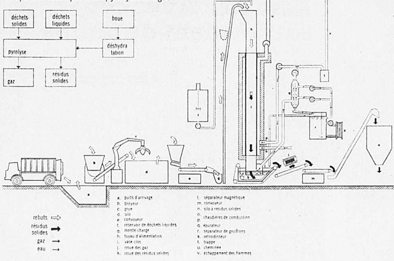
Coupe schématique d'un pyrolyseur à gaz
