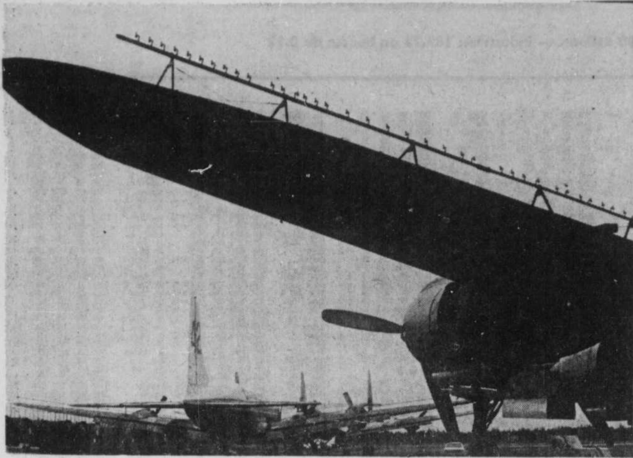
Sur les ailes des Super-Constellation qui faisaient la gloire des sociétés aériennes il y a 20 ans, on a posé des gicleurs savamment calibrés pour la pulvérisation des insecticides.
