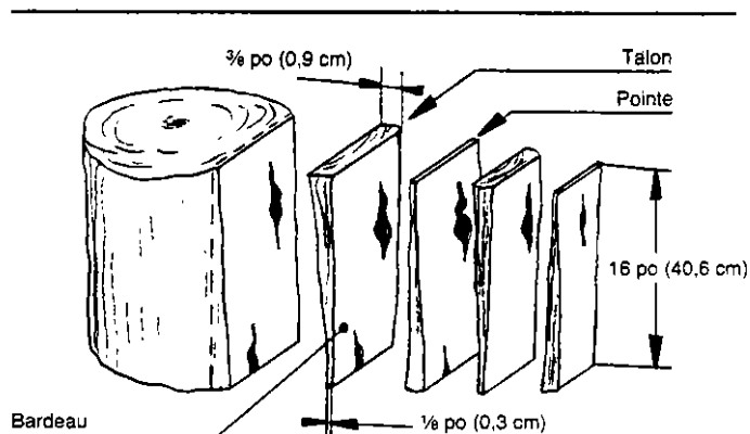
Figure 2: SCHÉMA DE COUPE DES BARDEAUX
