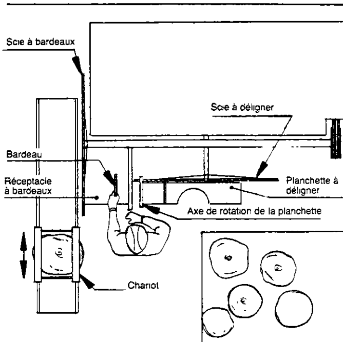
Figure 1: SCHÉMA DU POSTE DE TRAVAIL DE LA MACHINE À BARDEAUX
