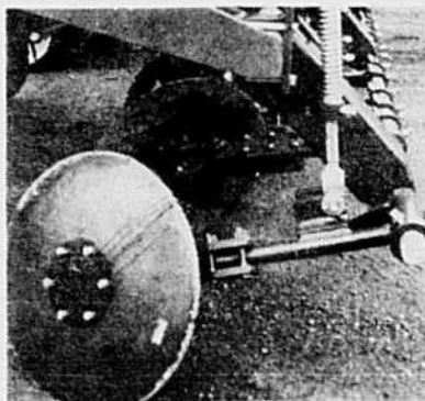
Préparateur à semis combiné avec semoir
