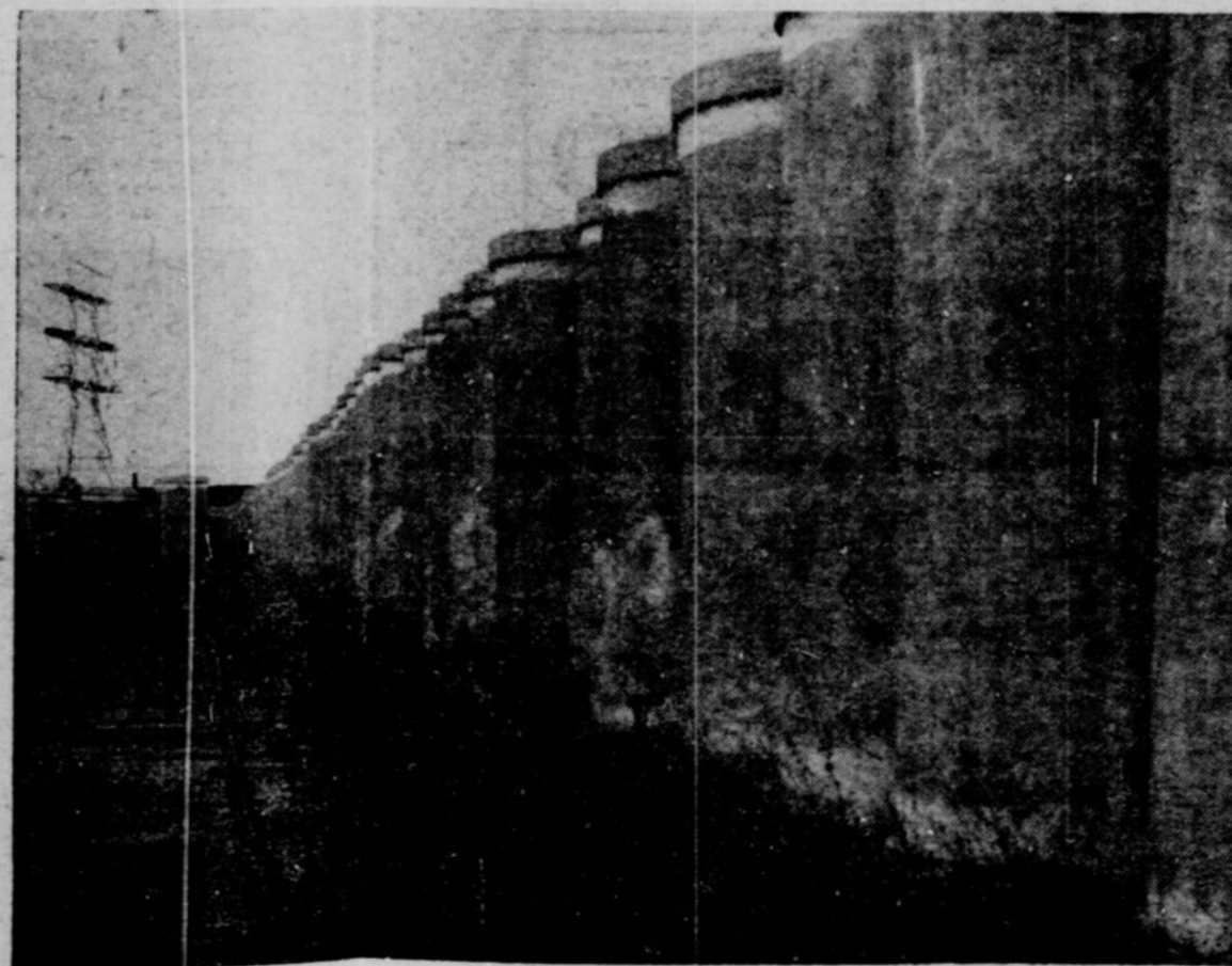
Une partie des tuyaux de sept pieds de diamètre qui serviront à la construction de la nouvelle prise d'eau verte provenant du lac Saint-Louis, plus pure que celle provenant de la rivière Outaouais, coulant près du rivage. Ces tuyaux coûtent à la ville environ $1,500,000, et l'on estime à autant le coût de la pose de ces tuyaux pour laquelle la ville de Montréal doit demander des soumissions prochainement.
