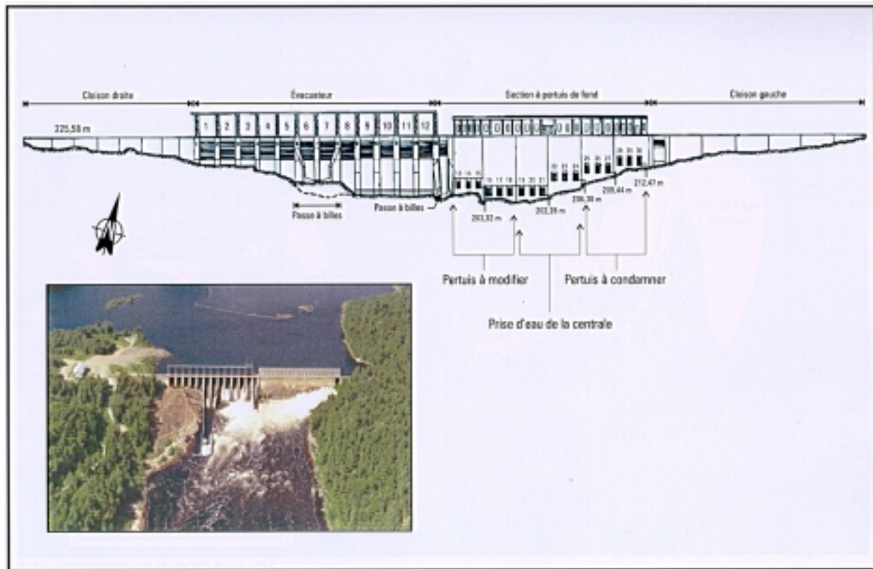
FIGURE 2 : CONFIGURATION DU BARRAGE MERCIER (TIRÉE DE L'ÉTUDE D'IMPACT)
