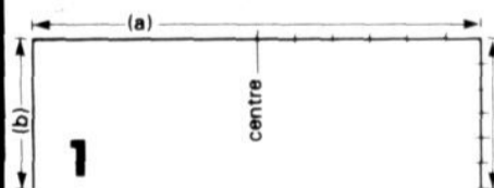
1.—tracer une largeur (a) et une hauteur (b), et marquer le centre de (a). Divisez en nombre égal de sections, la hauteur et la demi-largeur. Faire de même pour l'autre côté;
