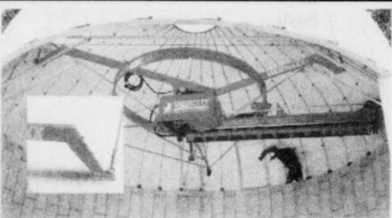
Bras de soutien incliné
