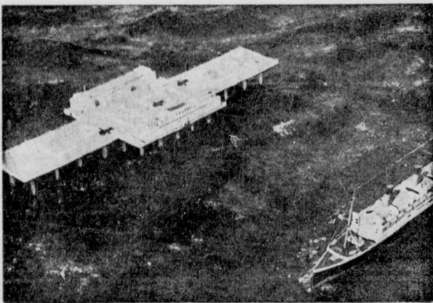
Un modèle d'aérodrome flottant au moyen duquel l'Atlantique pourrait être traversé dans de petits avions, par petites étapes.
