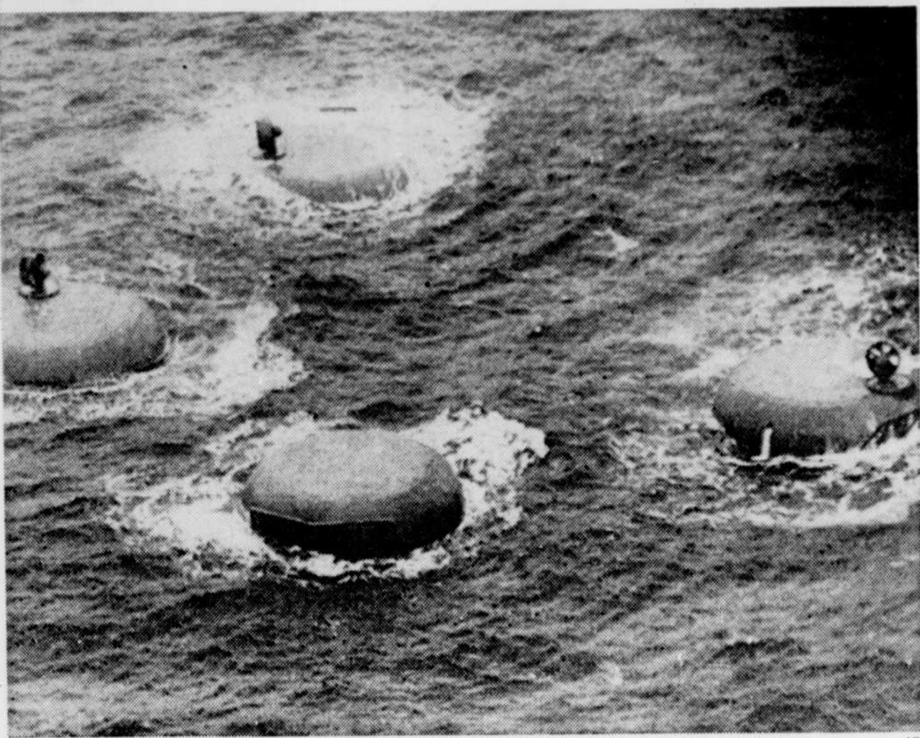
AP A vol d'oiseau, on ne voit plus que quatre des cinq pieds de la plate-forme pétrolière qui a chaviré jeudi soir en mer du Nord. Le cinquième pied s'est détaché et flotte dans le voisinage.
