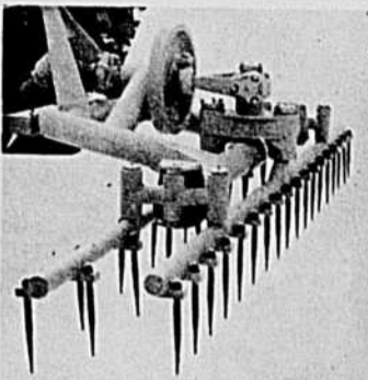
LA NOUVELLE HERSE À DENTS MOBILES FORANO
