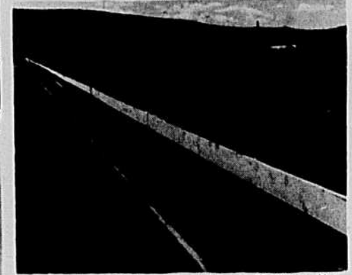
Mangeoire en béton monolithique, Medicine Hat, Alta; Van Read Mix Ltd.
