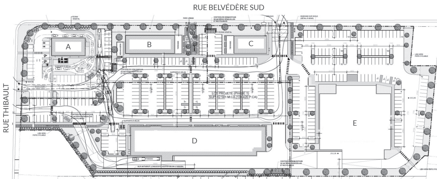
Implantation projetée des cinq bâtiments commerciaux situés rue Belvédère Sud.
