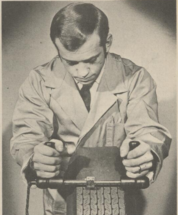
Bien que les pneus soient fabriqués en série dans des moules, on doit en construire et éprouver des prototypes individuellement. Dans le cadre de ce procédé, on doit découper à la main de nouveaux modèles de bandes de roulement, comme le fait ce dessinateur de l'usine de Goodyear-Canada à Toronto, à l'aide d'un couteau chauffé électriquement qui pénètre aisément dans le caoutchouc.
