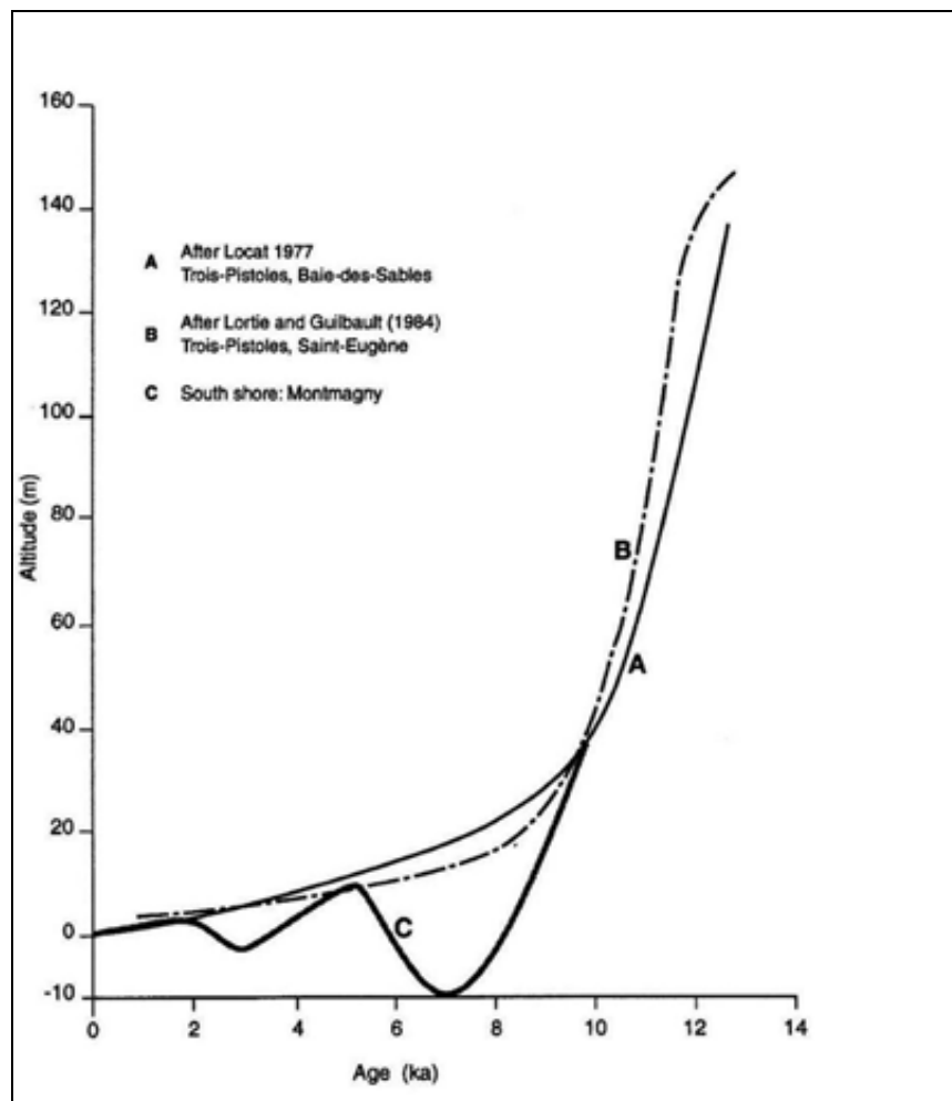
Figure 2 : Courbe d'émergence des terres dans l'estuaire du Saint-Laurent (Dionne 1988 : 241).
