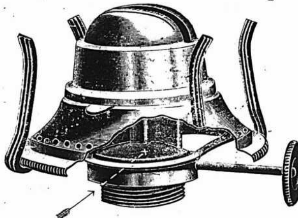
Brûleur Banner pour Kérosène.
