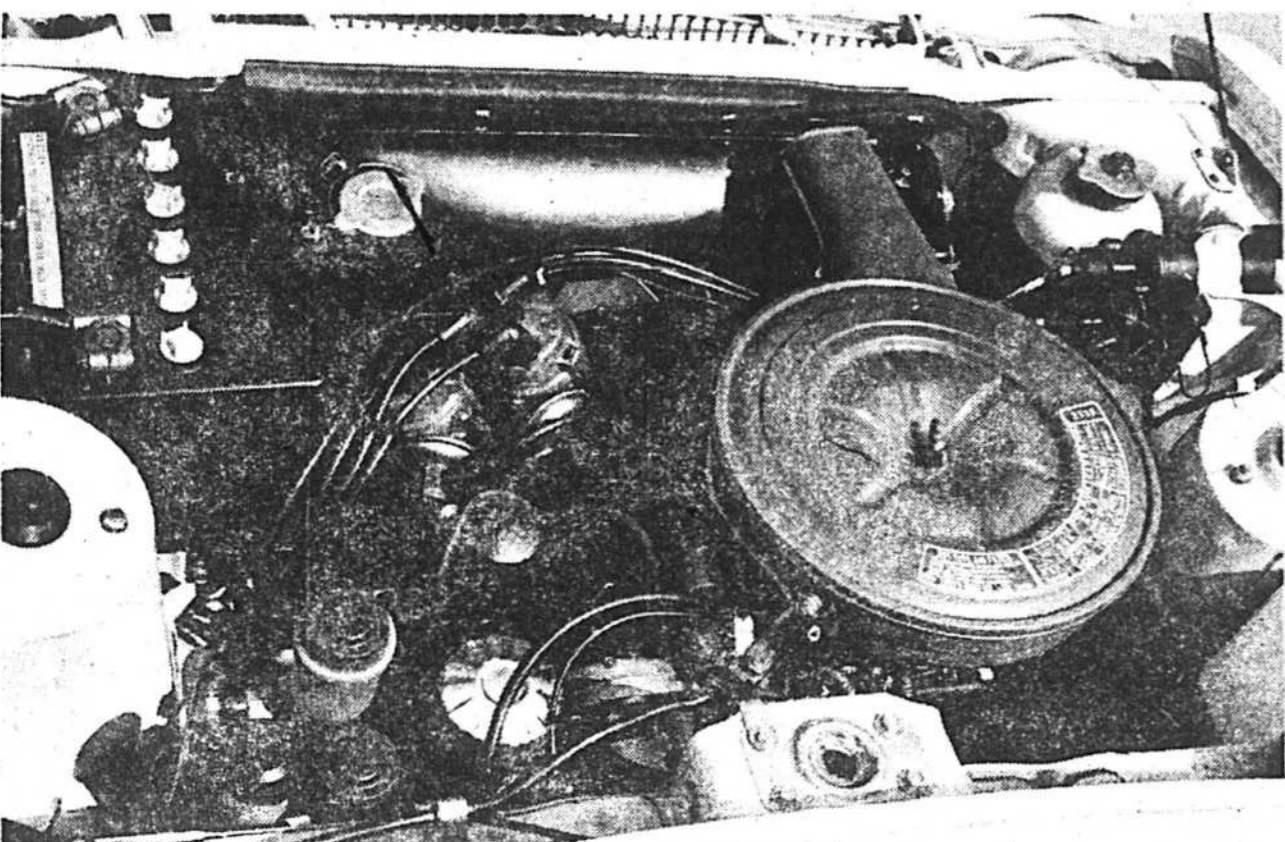
Voici le moteur rotatif à deux rotors qui équipe la nouvelle Mazda R-100. On remarquera les deux bobines à droite et les deux distributeurs au centre. Sous le capot, les acces-
