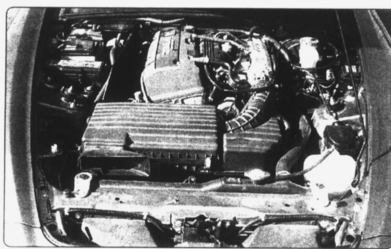
Le moteur de la S2000 est un 4 cylindres VTEC de 2,0 litres multisoupape à double arbre à cames en tête de 240 chevaux dont la ligne rouge se situe à 9 000 tr/mn.
