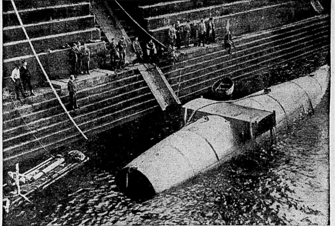
LA NAVIGATION AERIEENNE — Ce qui semble une gondole dernier cri ou un sous-marin nouveau genre n'est en réalité qu'une section de l'"Ambassador", un avion britannique à passagers, alors qu'il subit les tests d'imperméabilité habituels, à Southampton, G.-B. On vérifie ainsi la solidité de construction du fuselage et de la partie centrale de l'appareil. Vingt de ces aérobus seront bientôt mis en service par différentes compagnies aériennes anglaises.
