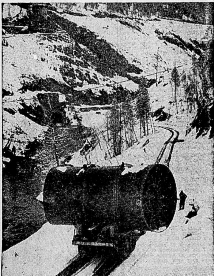
GIGANTESQUES INSTALLATIONS — La tâche d'installer les sections des énormes tuyaux du "Hungry Horse Project", au Montana, comporte, comme on le voit, certaines difficultés. Ici, une de ces sections de vingt pieds de longueur et de vingt tonnes est descendue vers le barrage où elle sera soudée. Environ 1,800 pieds de tuyauterie seront enfouis dans la digue d'une hauteur de 564 pieds, et permettront de conduire l'eau vers quatre immenses turbines.
