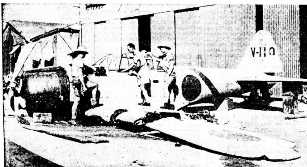
Un avion de chasse japonais Zéro a été abattu, près de Port Moresby, en Nouvelle-Guinée. Il a été transporté au terrain d'aviation où des pilotes américains et australiens en font un examen approfondi.
