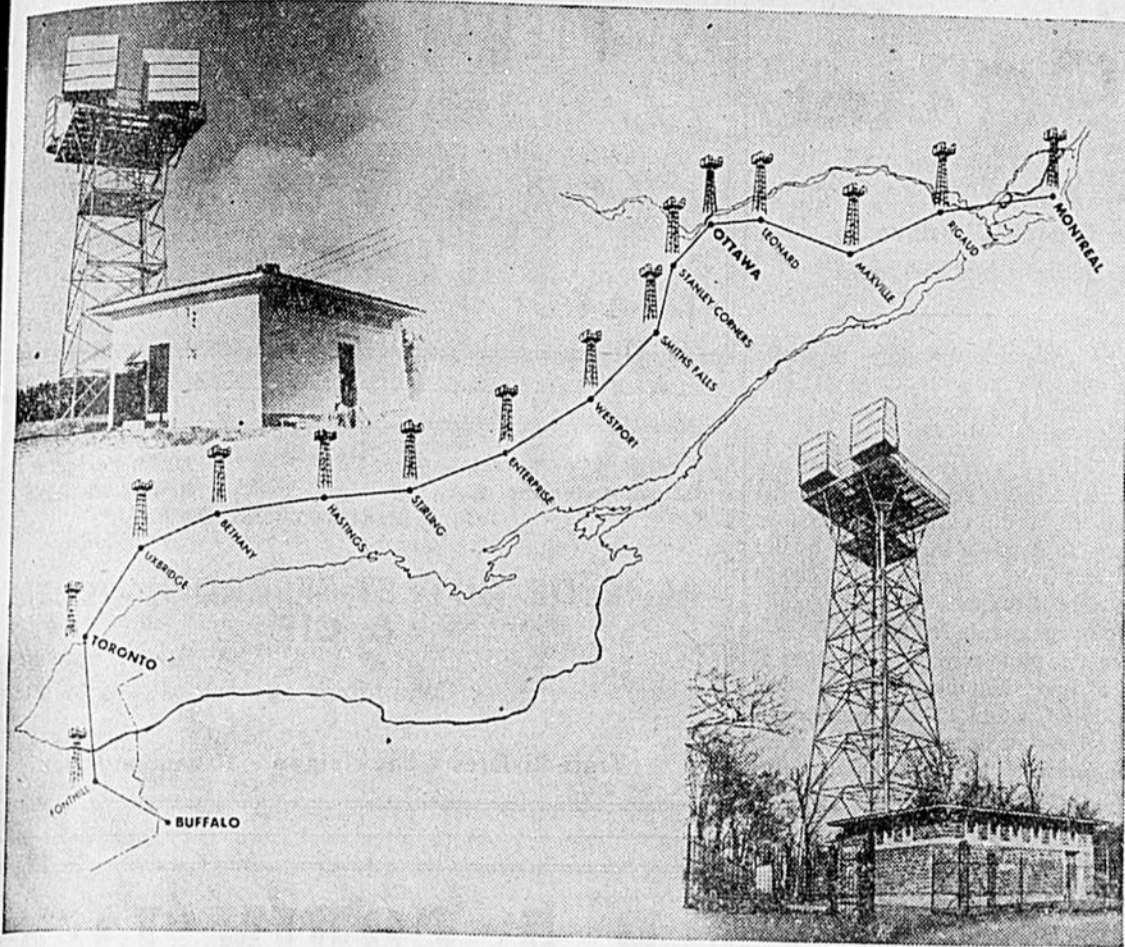
Carte du réseau de télévision de Radio-Canada avec ses relais à ondes micrométriques qui ont été érigés par la Compagnie de téléphone Bell. En bas, à droite, le pylône terminus de Montréal, qui a été érigé sur le mont Royal. On aperçoit à l'arrière-plan l'antenne de CBFT. En haut, à gauche, l'une des 13 stations de relais entre Montréal, Ottawa et Toronto.
