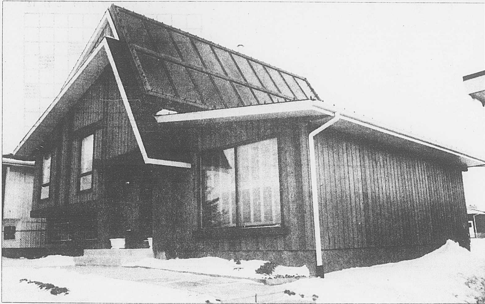
Cette maison solaire, de modèle conventionnel avec toit modifié, a été construite par Nu-Est Corporation, et sert de maison-modèle dans une banlieue de Calgary. Le système solaire a été conçu pour répondre à 80 pour cent des besoins annuels de la
