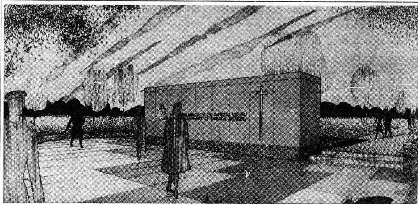
MONUMENT COMMEMORATIF — Ce magnifique monument qui sera érigé dans le parc Major rappellera les 1,886 hommes de l'Artillerie royale canadienne qui ont donné leur vie au cours du second conflit mondial. Le monument occupera un emplacement d'environ 75 pieds carrés. Il aura 31 pieds de longueur et huit pieds de hauteur, le
