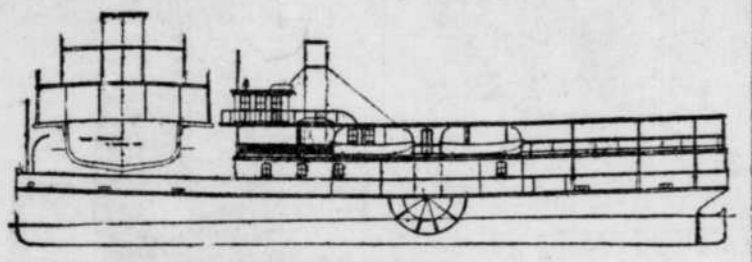
Le plan du nouveau traversier le "Gérard" qui fera le service entre Montréal et l'île Sainte-Hélène.
