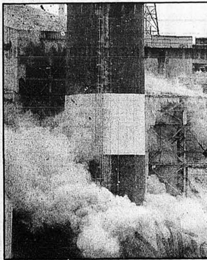
Derrières vérifications avant l'explosion: tout semble prêt, on y va. Mais quand la poussière retombe, la deuxième cheminée, amputée de cinq mètres, est toujours debout.
