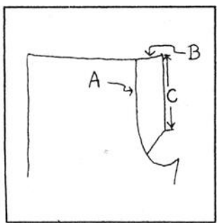
A. Ligne de coupe normale B. Prolonger 1 1/4" C. Glissière
