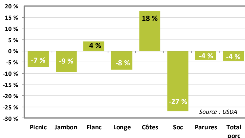
Variation des quantités de porc en entreposage frigorifique aux États-Unis, juillet 2018 par rapport à la moyenne 5 ans (2013-17)
