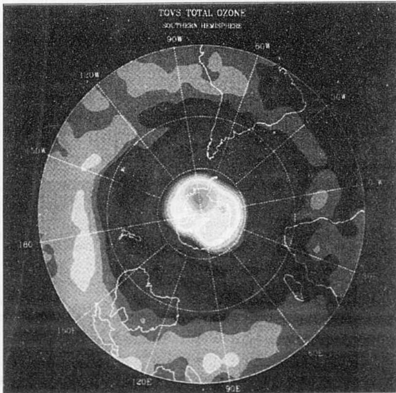
Représentation graphique de la détérioration de la couche d'ozone au-dessus de l'Antarctique en 1992.
