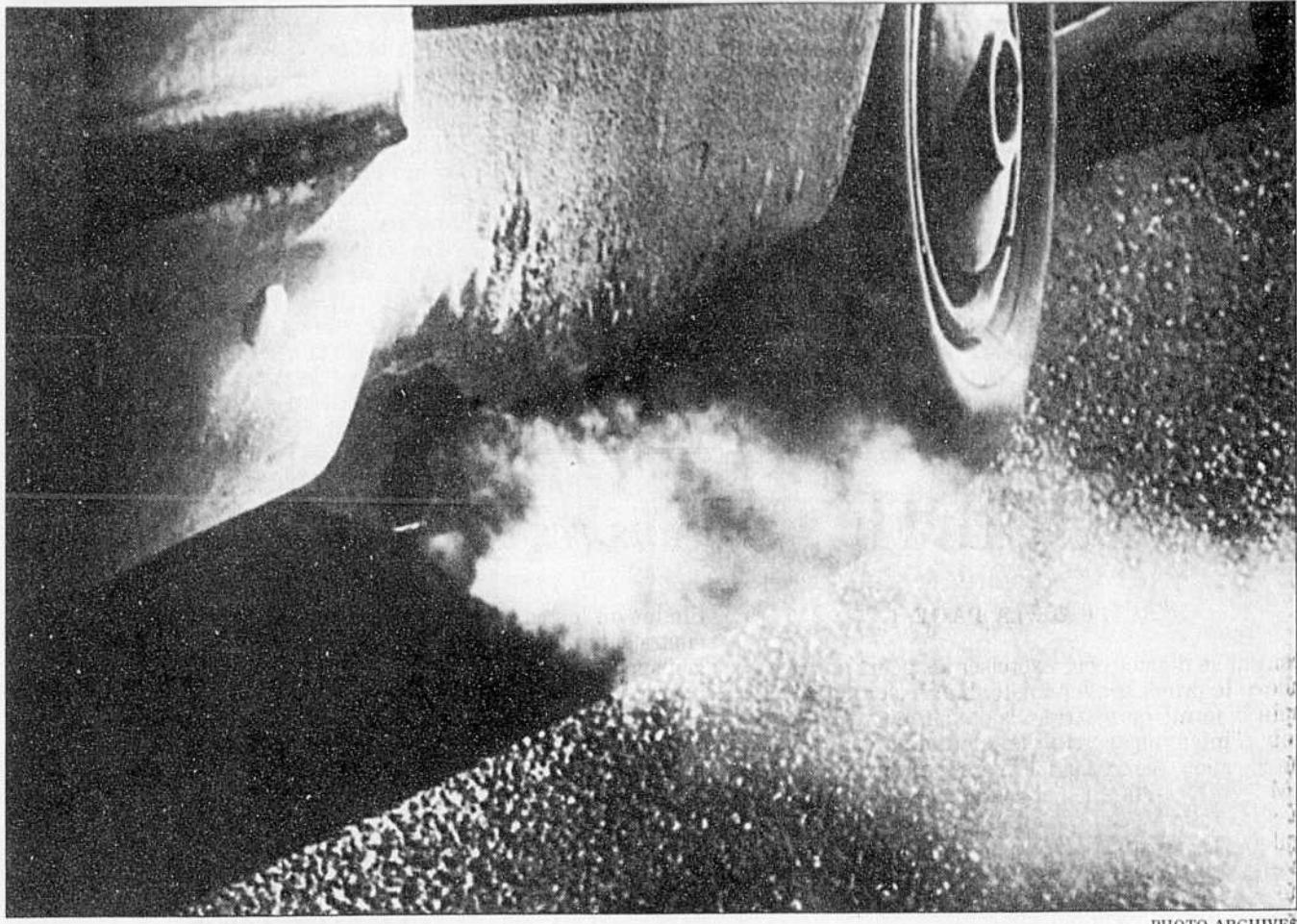
Les combustibles fossiles (pétrole et charbon), en brûlant, dégagent chaque année quelque 5,5 milliards de tonnes de gaz carbonique.
